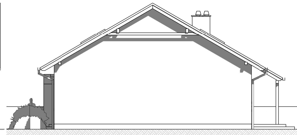
Elewacja zachodnia
