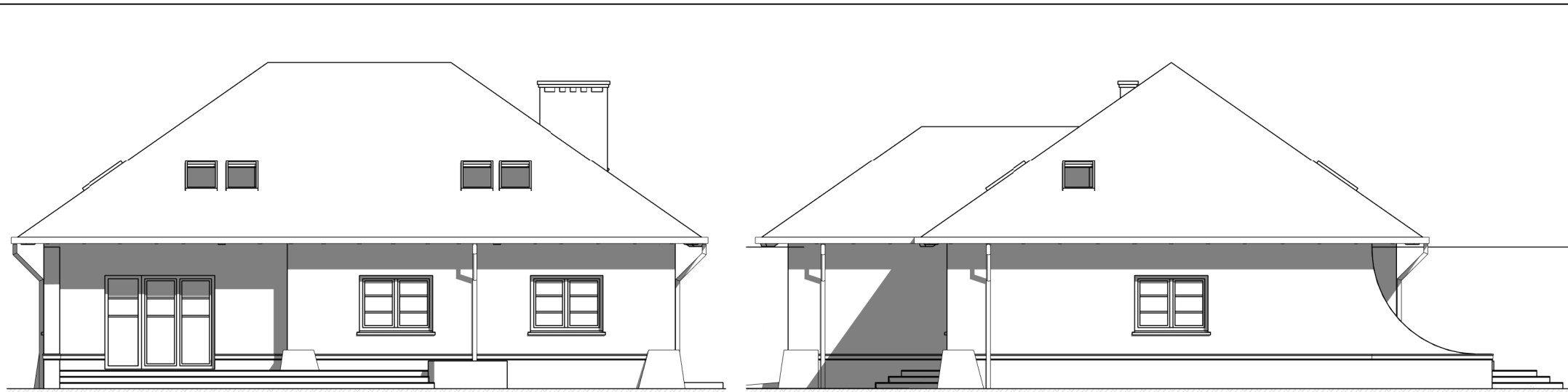
Elewacja południowa
