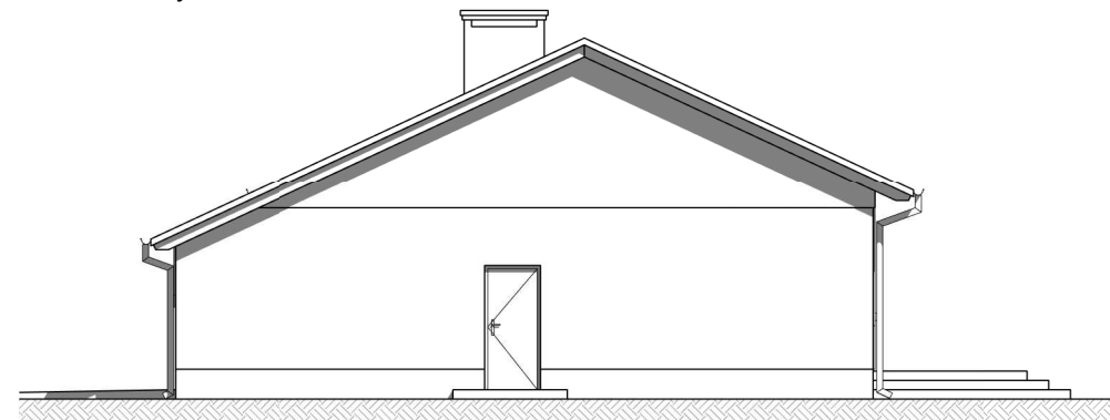
Elewacja zachodnia
