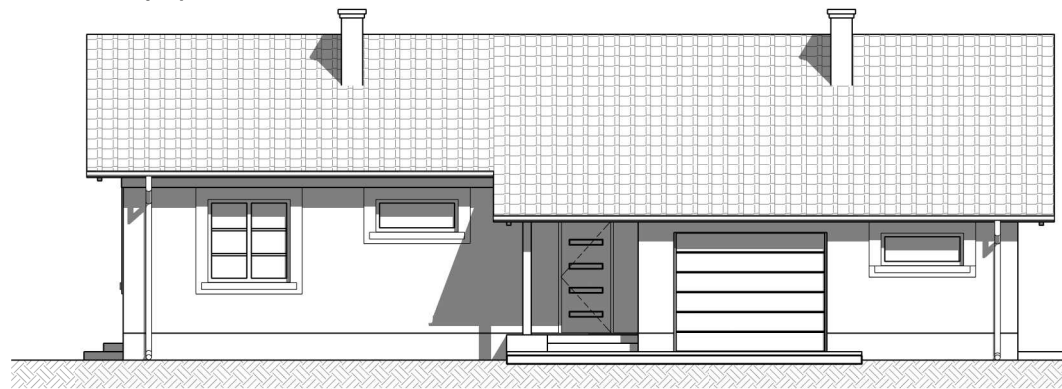
Elewacja południowa
