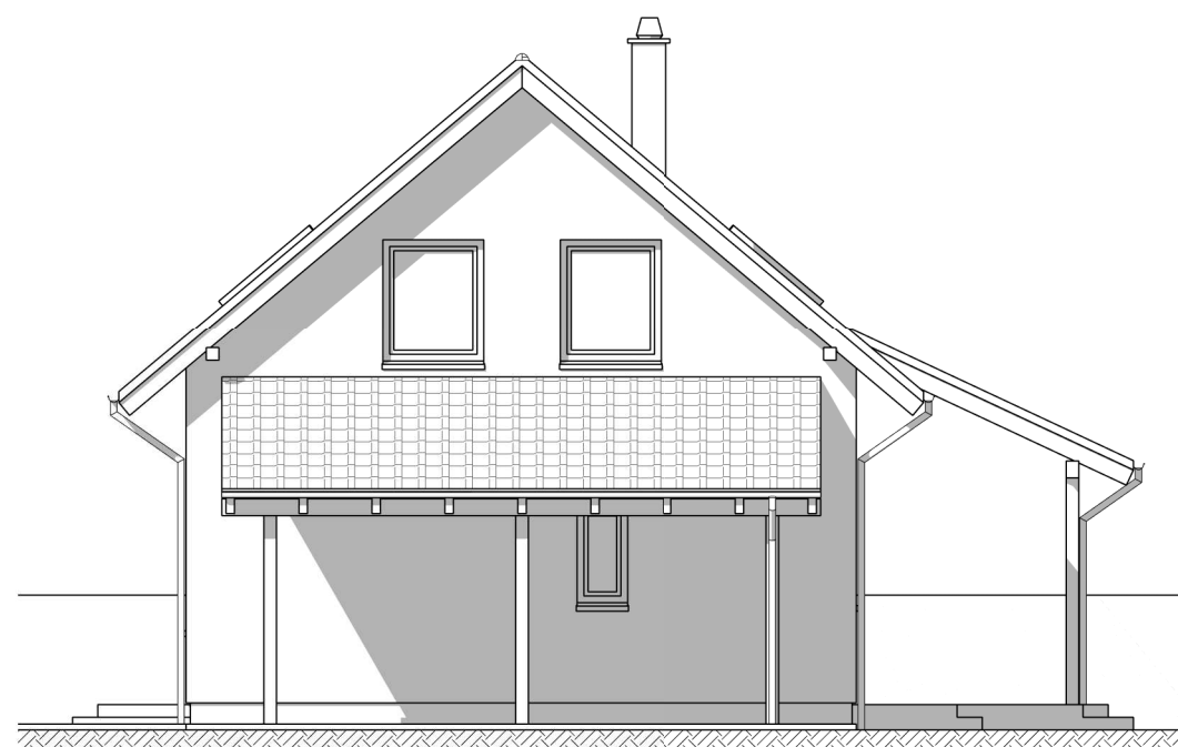
elewacja wschodnia
