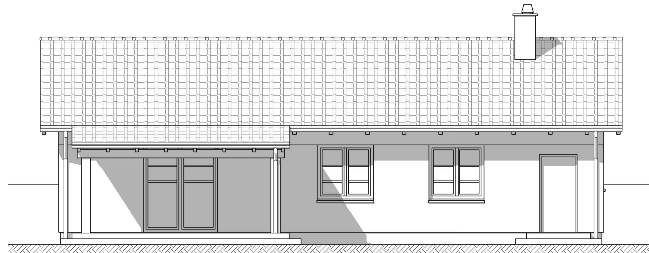
elewacja północna
