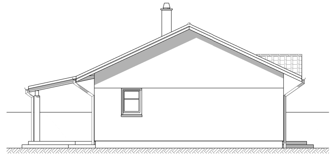
elewacja zachodnia
