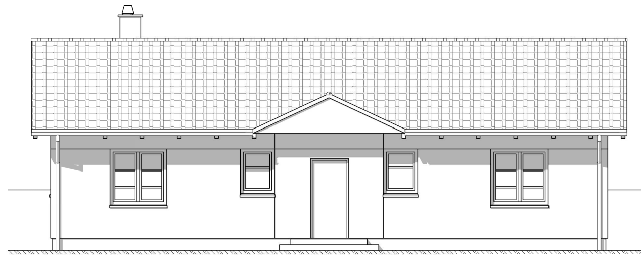
elewacja południowa
