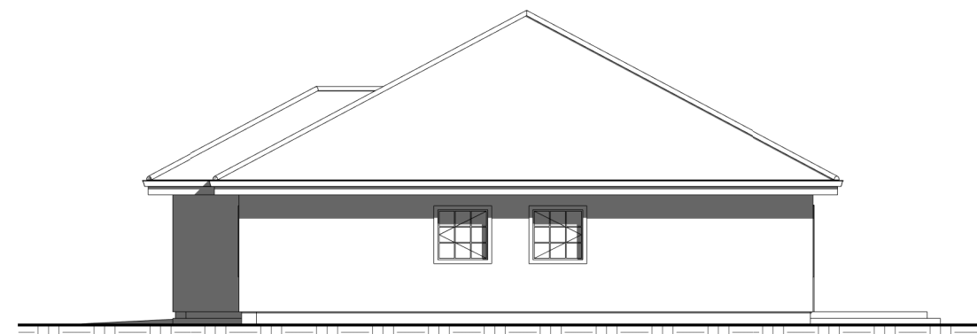
ELEWACJA WSCHODNIA
