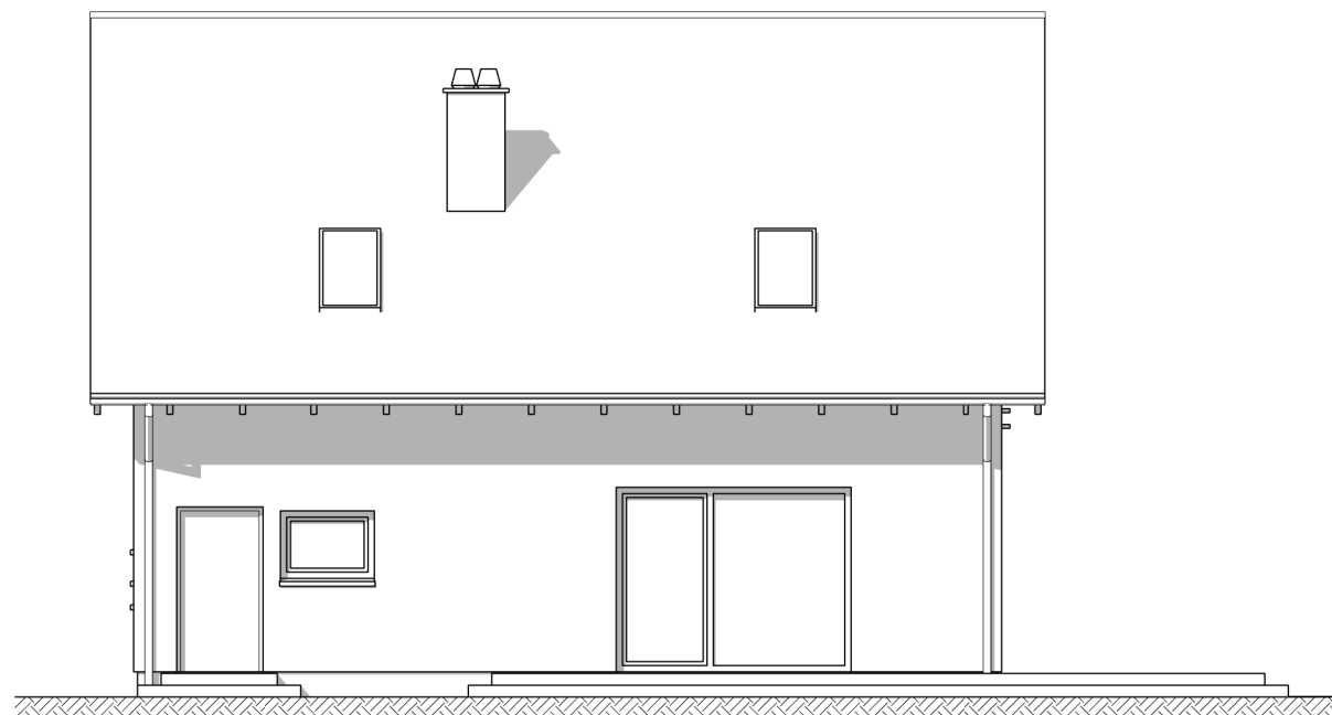
elewacja południowa
