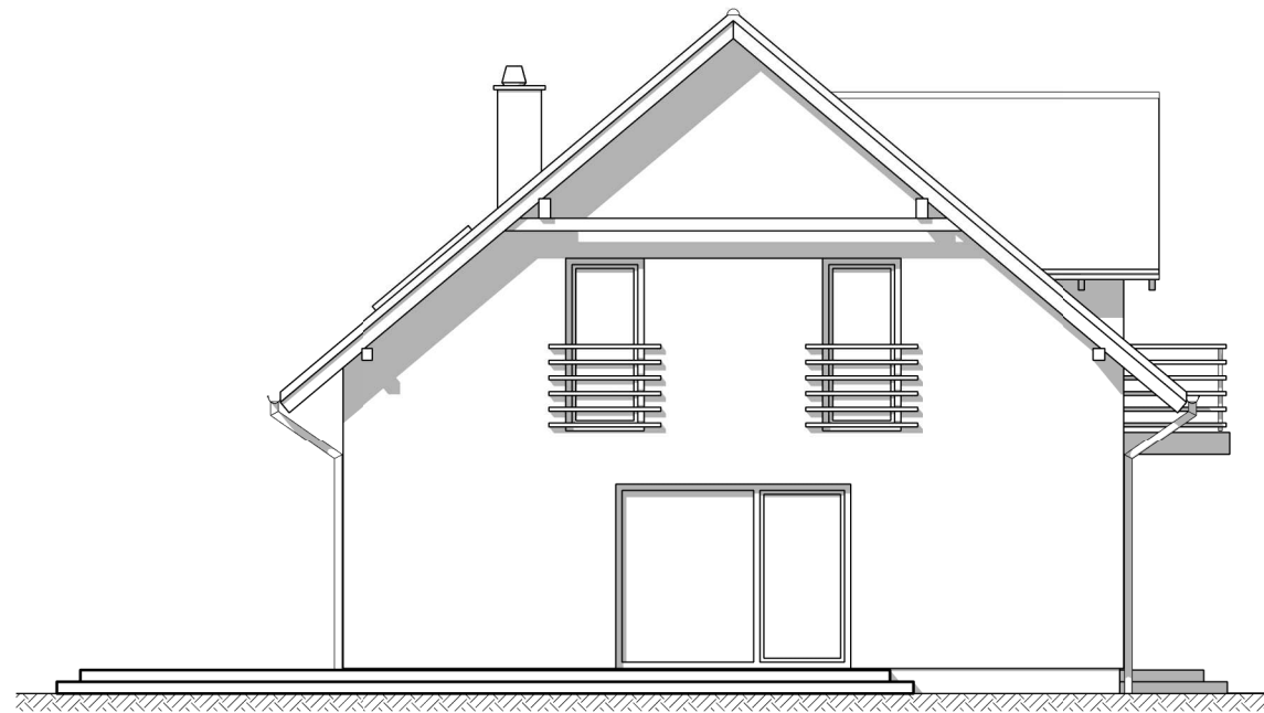
elewacja wschodnia
