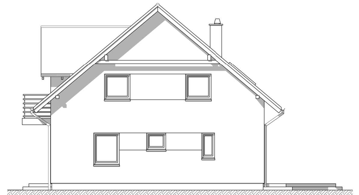
elewacja zachodnia
