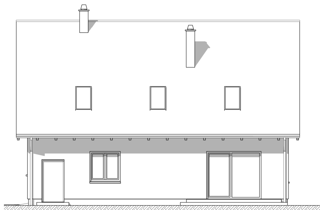
elewacja zachodnia
